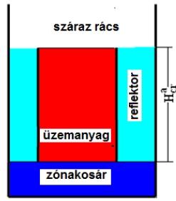
4.b. ábra: A mérés axiális rajza a korrekció után, távtartó rács nélkül
