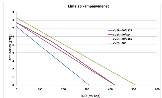
9. ábra. VVER reaktorok elméleti kampánymenetei
