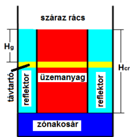
4.a. ábra: A ZR-6 sematikus elrendezése a távtartó ráccsal
